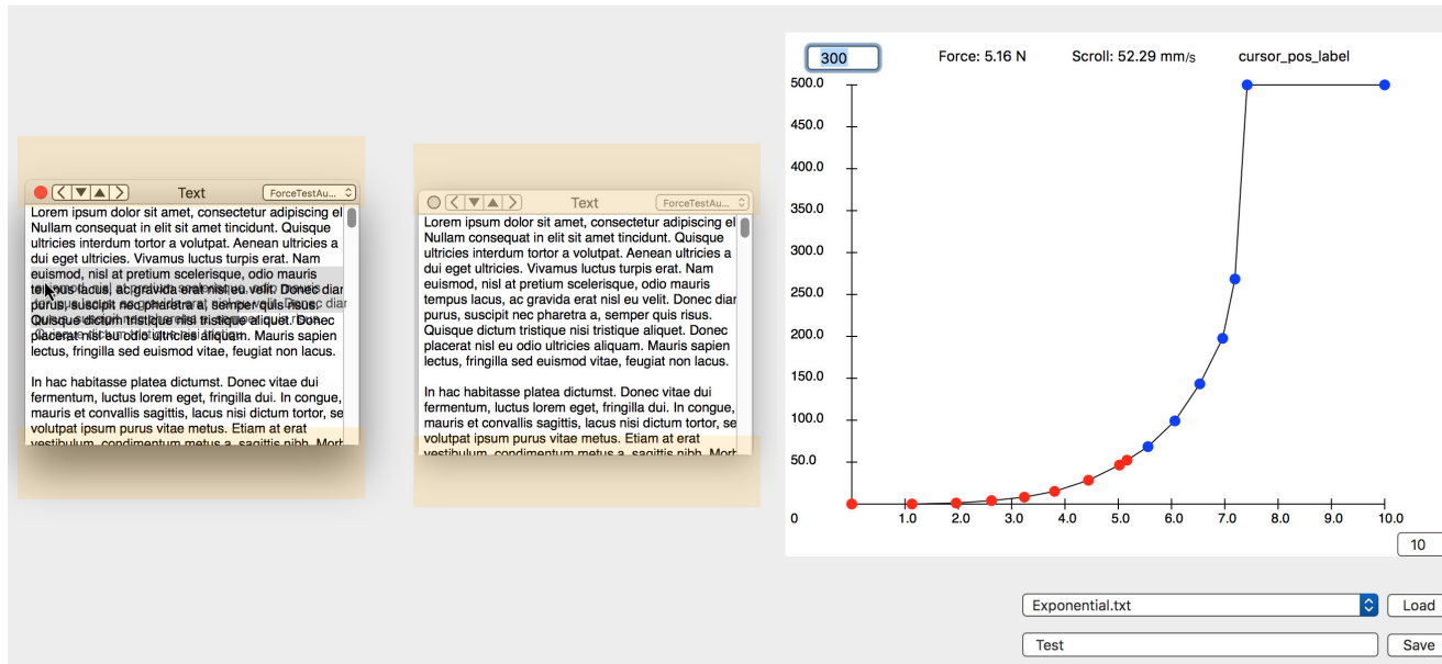
Figure 2: Démonstrateur mettant en oeuvre ForceEdge. Il permet de créer plusieurs vues (ici 2) supportant l'autoscroll via ForceEdge. Le diagramme situé à droite permet de modifier la fonction de transfert convertissant la force exercée sur le pavé tactile en vitesse de défilement.
